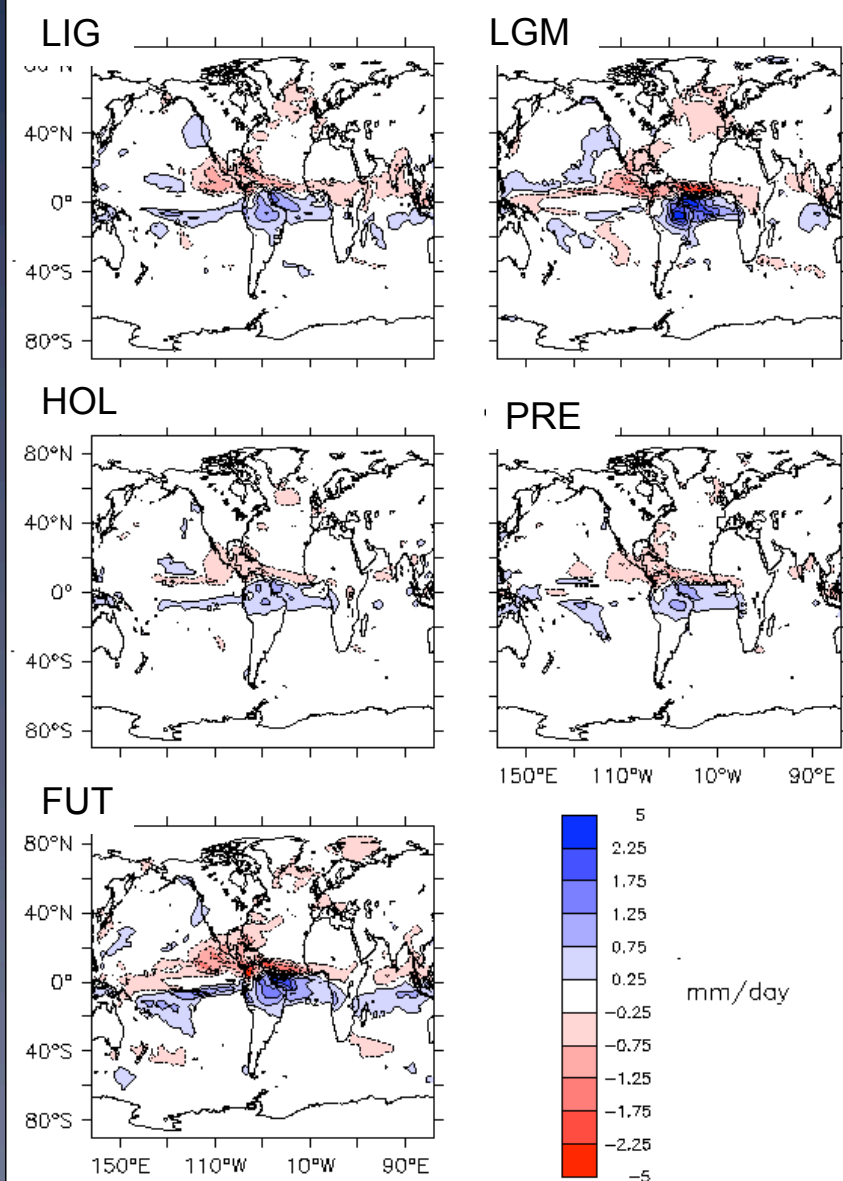
Précipitation
