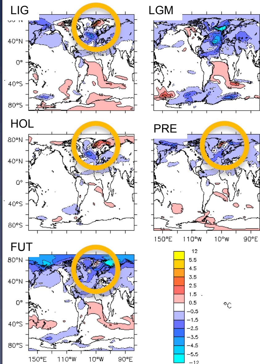
Température
